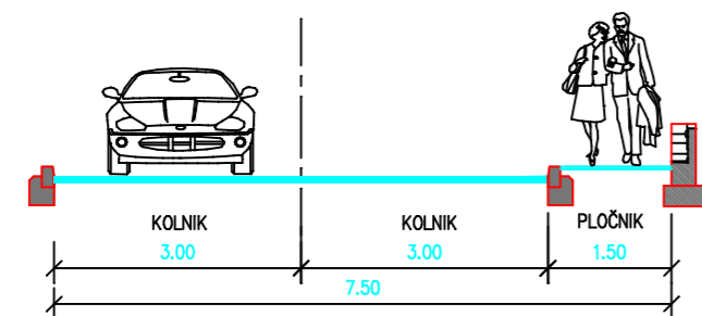
PROFIL TIP C
