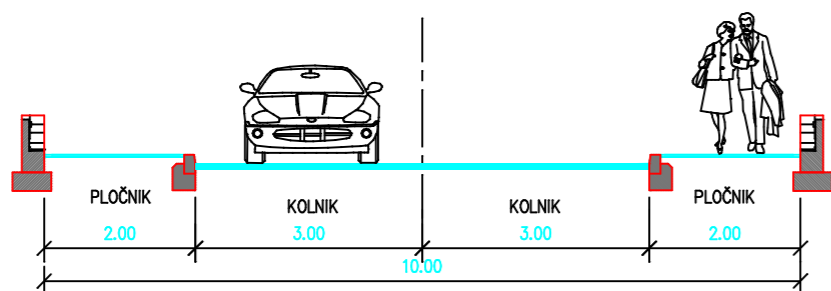
PROFIL TIP A
