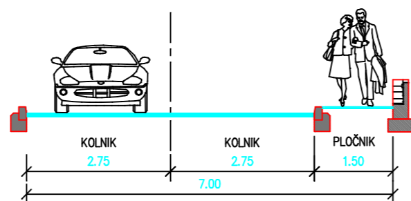
PROFIL TIP D
