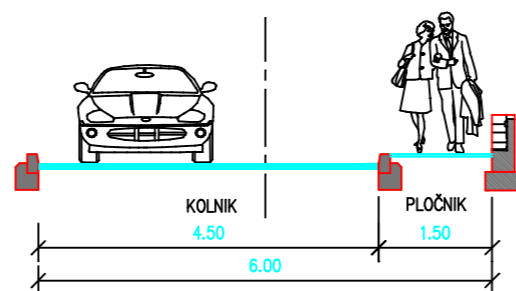
PROFIL TIP E
